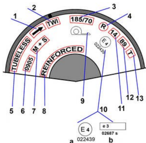
Figura 25 – Codici dello pneumatico
